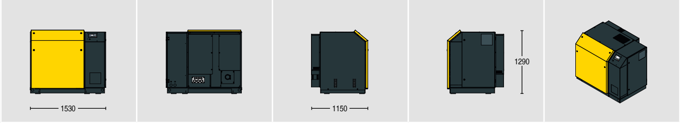
Серия СВ 166/236 С – без распределительного шкафа
